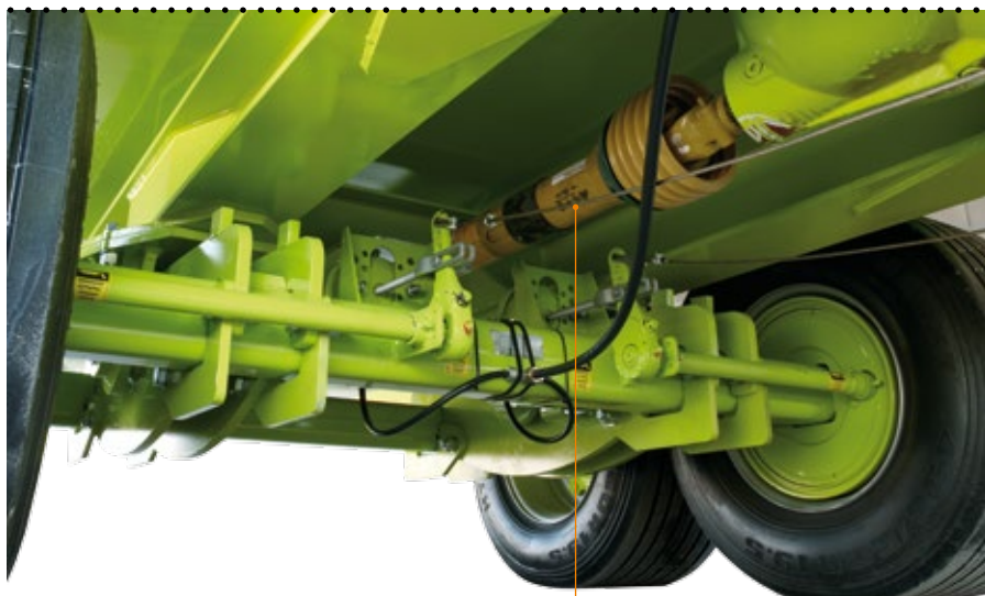
Cardani per impieghi gravosi Heavy duty PTO shaft
